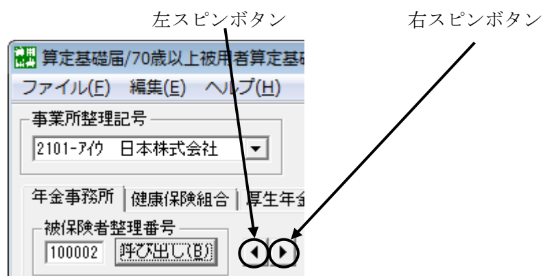
図 5-57. スピントン
