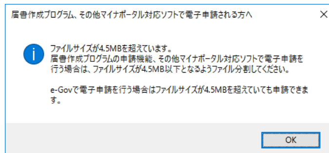
図3－1－1. 確認画面
