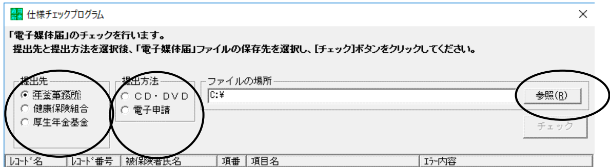
図3-1. メイン画面
