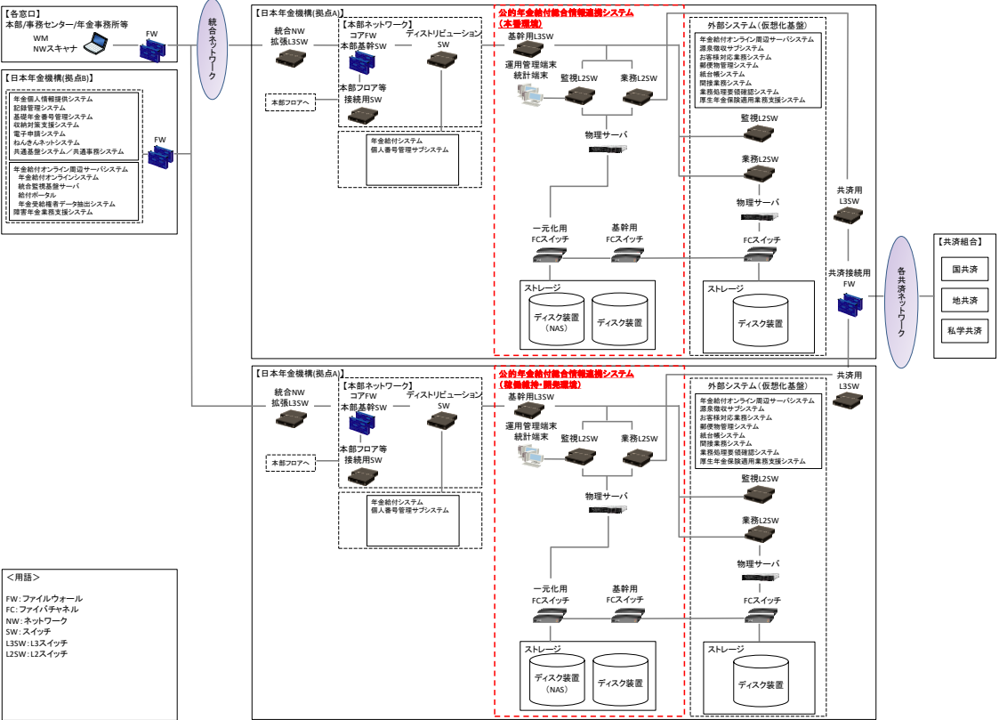
図 4.2.2-1 システム全体構成
